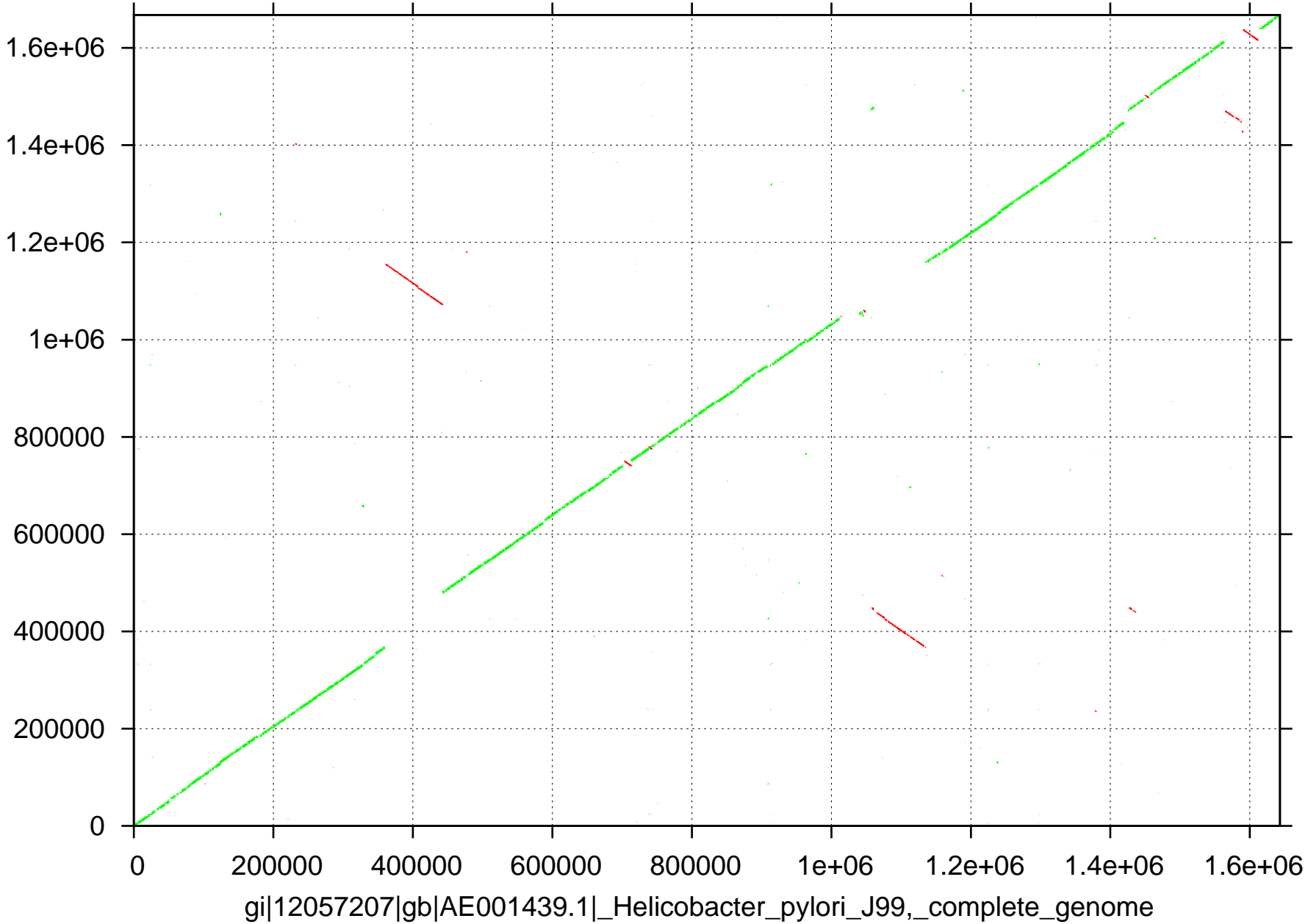
plot_matches
